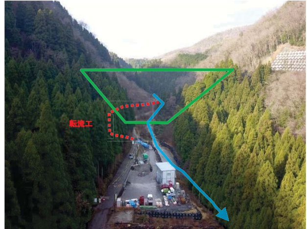
【転流工：吉野瀬川ダム（1,280百万円）】
