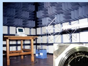
電波暗室
