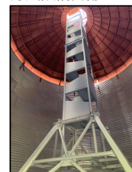
貯蔵設備内部
