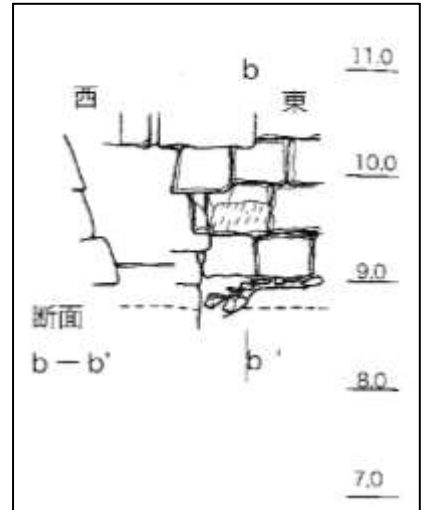
トレンチE立面図
