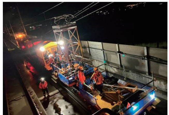
模擬パンタグラフを用いた電車線測定の様子
