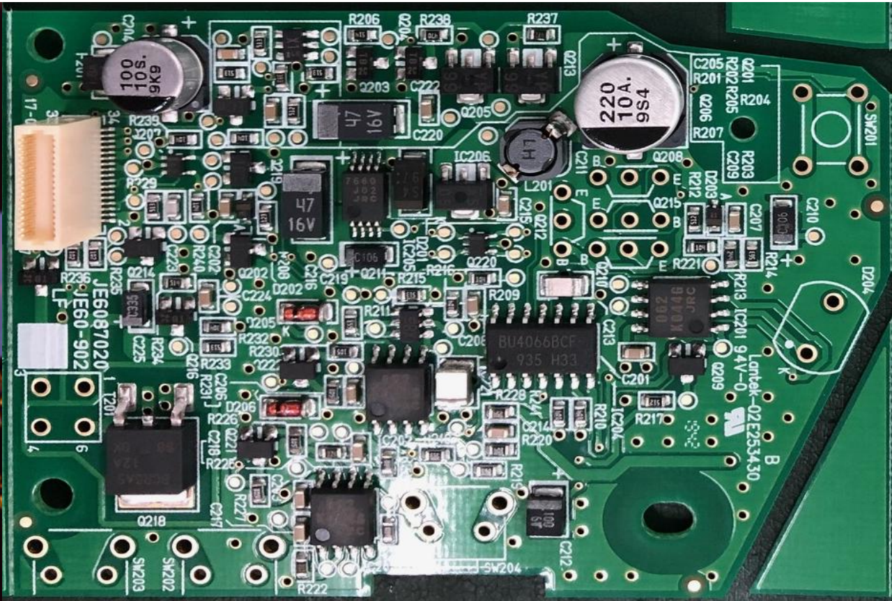
ヘッドアップディスプレイ用基板 Circuit board for head-up display
