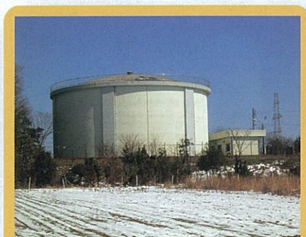
②あわら市第2県水受水場 (4,000m 3 )
