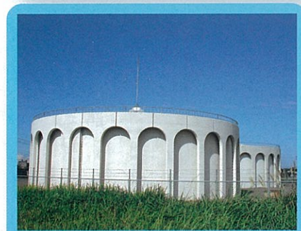
⑥坂井市坂井上水道管理センター (1,100m 3 ×2池)
