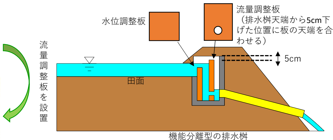
「田んぼダム」を実施している水田のイメージ
