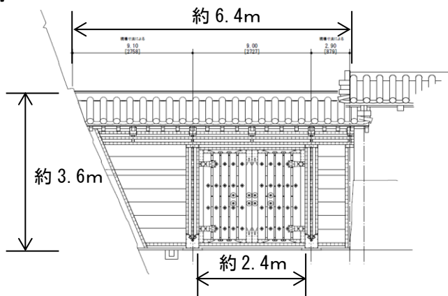
立面図（正面、北側）
