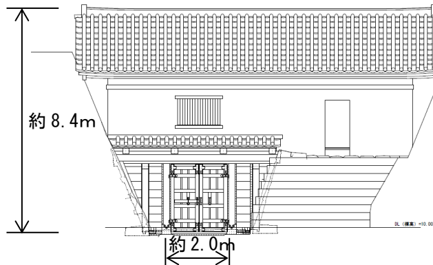
立面図（東側（県庁側））
