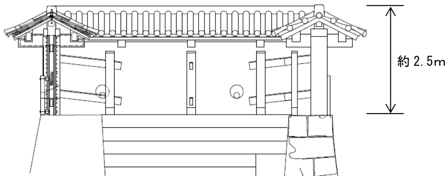
立面図（東側、枡形石垣内）
