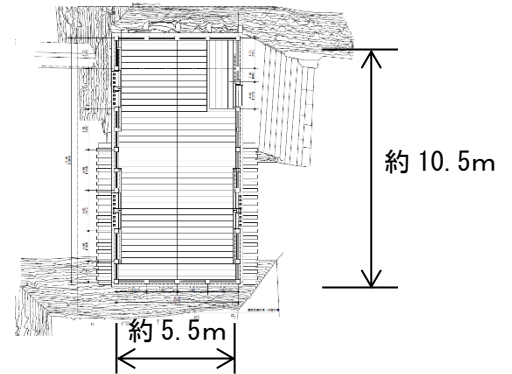
平面図（2階）
