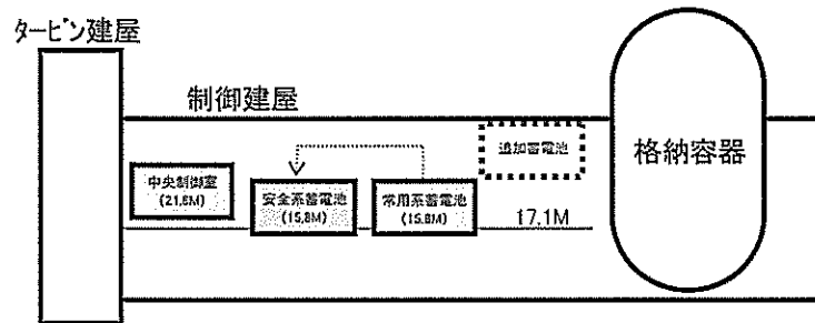
大飯3,4号機蓄電池配置イメージ図
