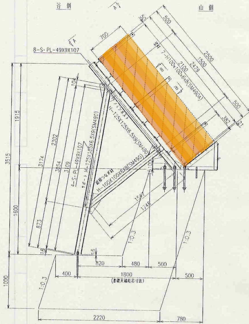
断面図 1/20
