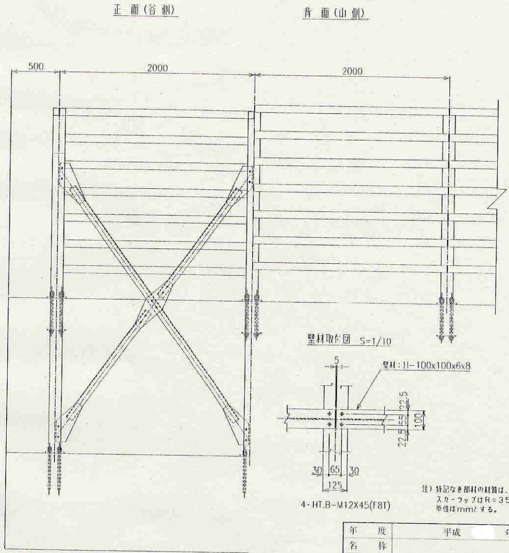
正面図 1/20
