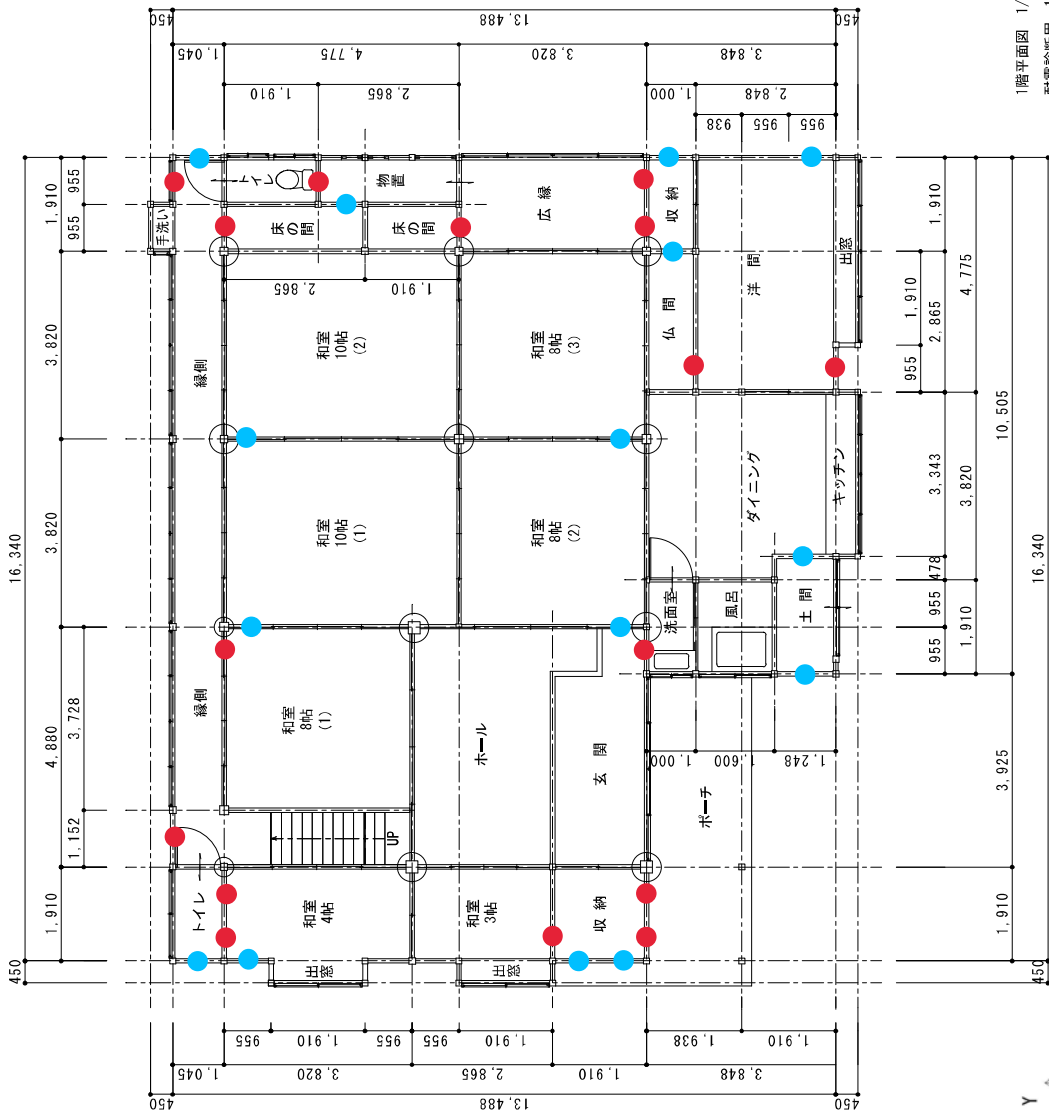
1階制震ダンパー設置計画図 S=1/100
