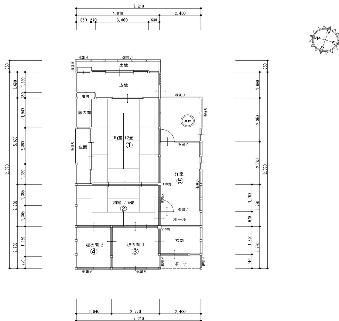
1 階平面図
