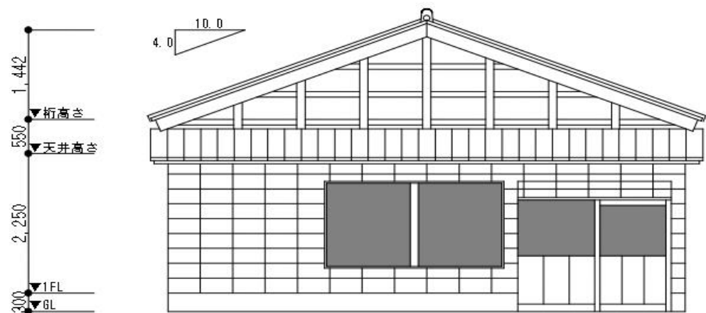
南側立面図
