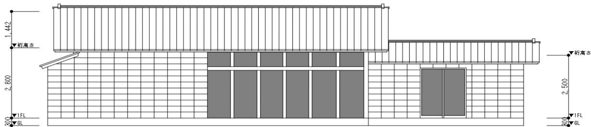
東側立面図
