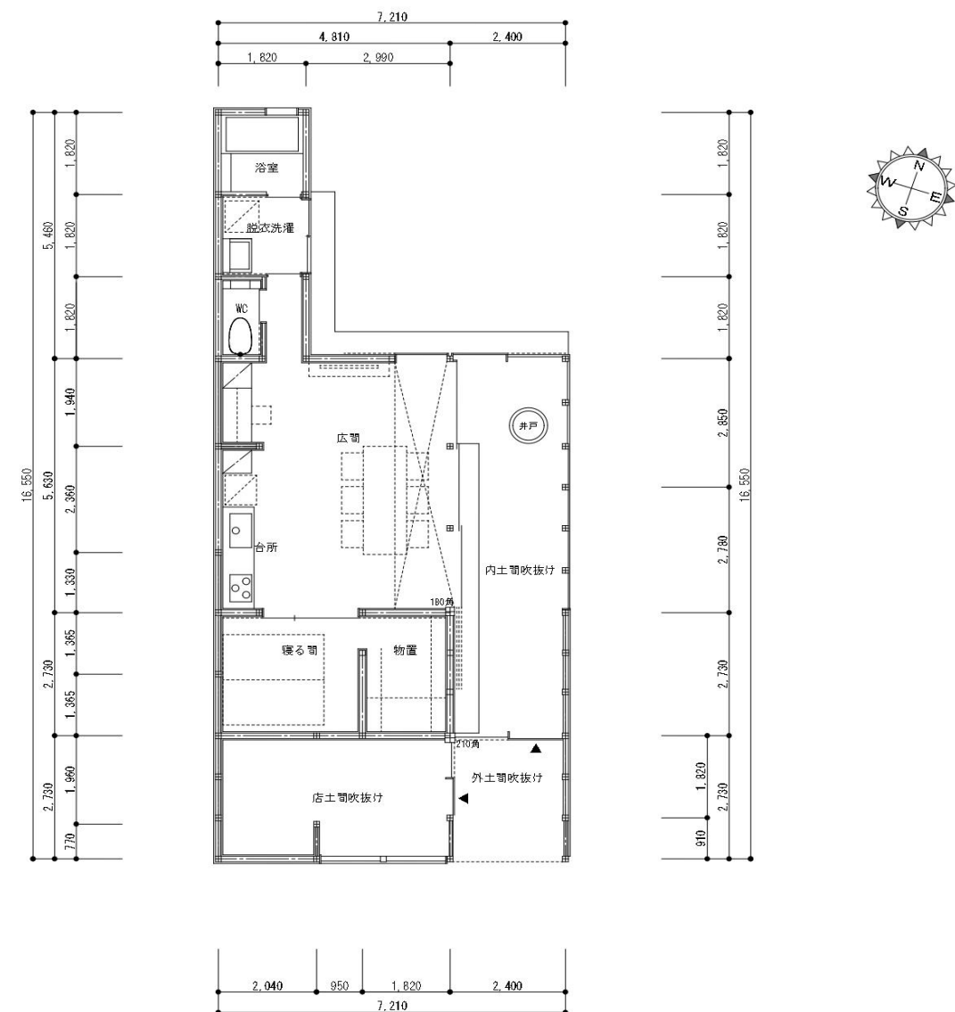
1 階平面図
