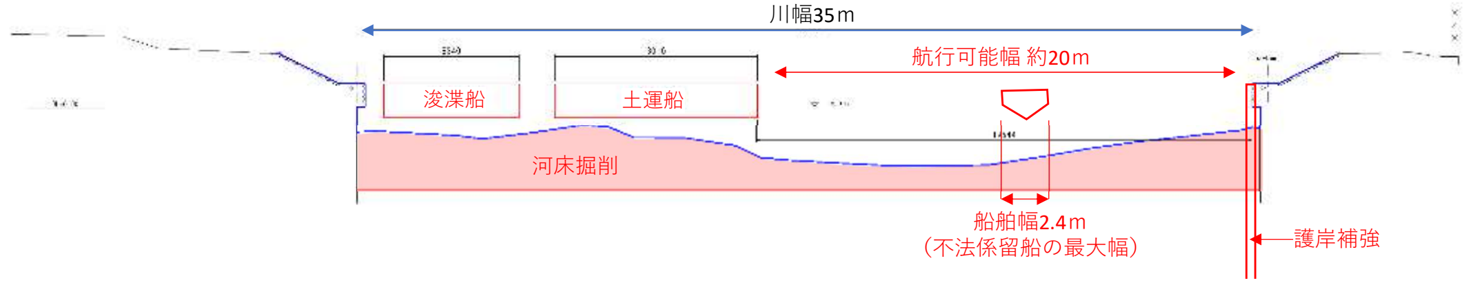
櫛川工区標準横断面図
