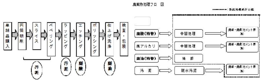
福井工場工程図
