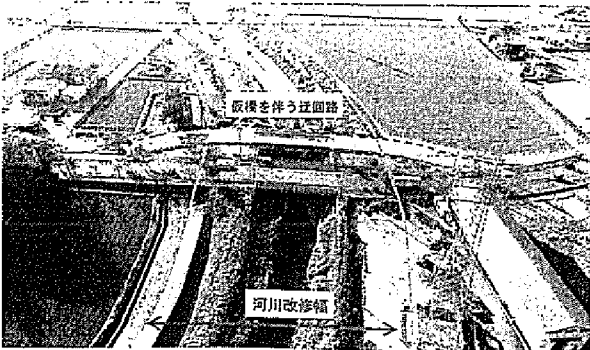
河道拡幅工事 芦原街道(新橋) 令和4年11月撮影
