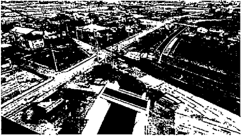
完成した市道橋(手前)とえちぜん鉄道の仮線路敷設工事(北川:春江町針原) 令和元年12月10日撮影
