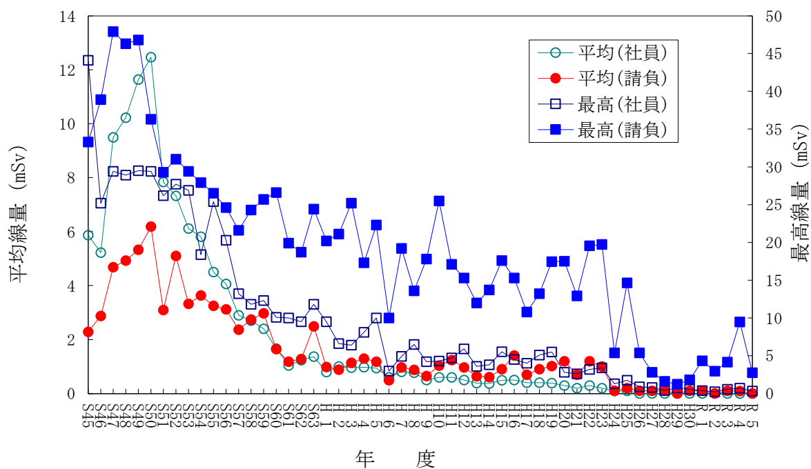
敦賀発電所従事者 平均・最高線量
