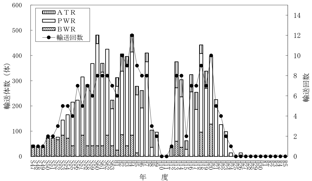
使用済燃料の輸送実績（県内発電所合計）
