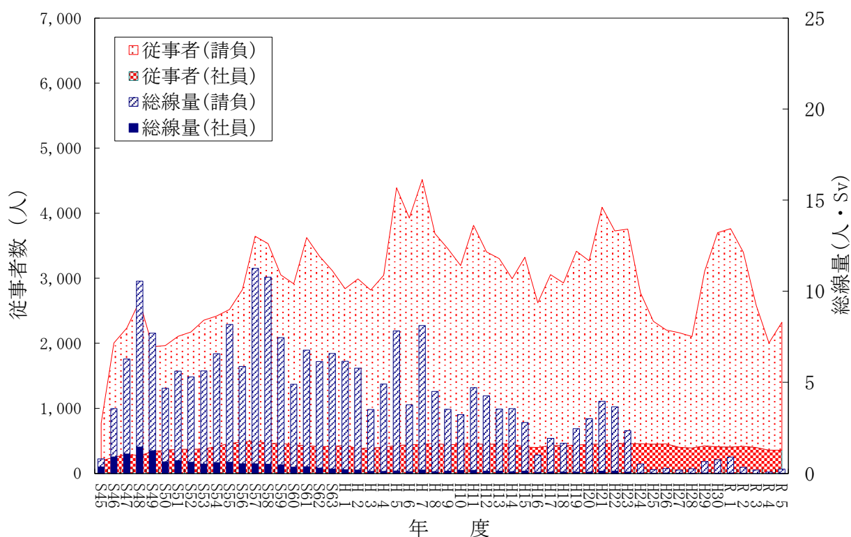
美浜発電所 従事者数・総線量
