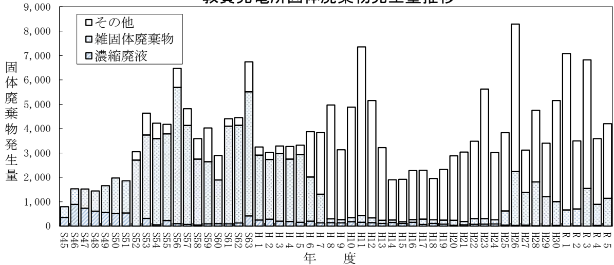
敦賀発電所固体廃棄物発生量推移
