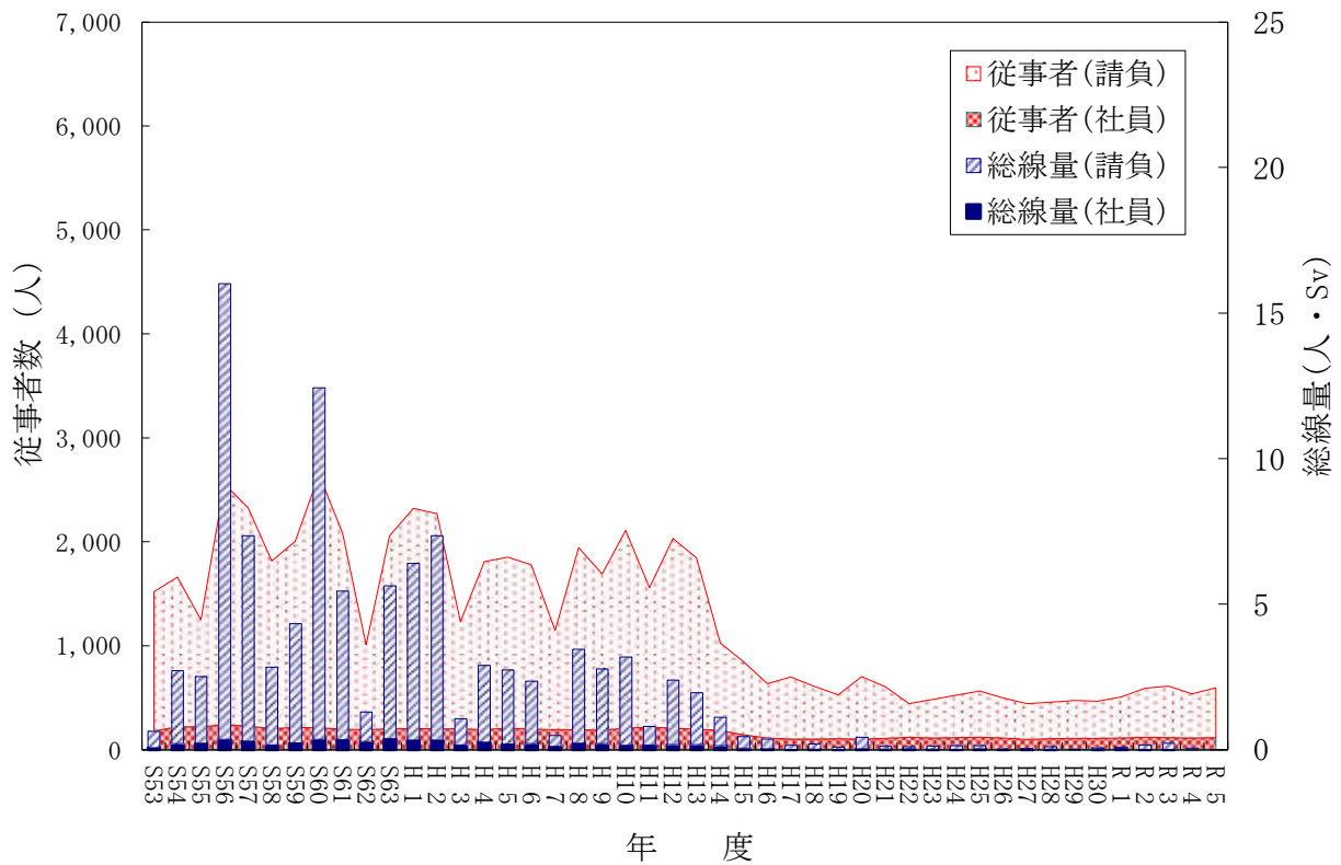
新型転換炉原型炉ふげん従事者数・総線量
