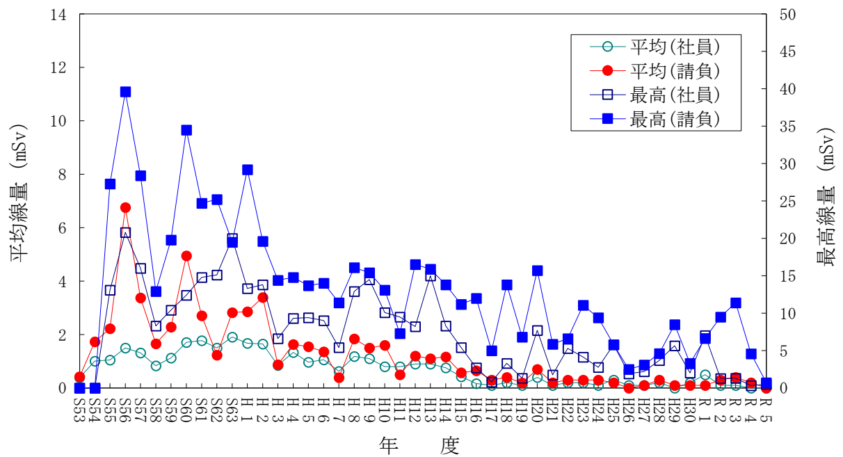
新型転換炉原型炉ふげん従事者 平均・最高線量
