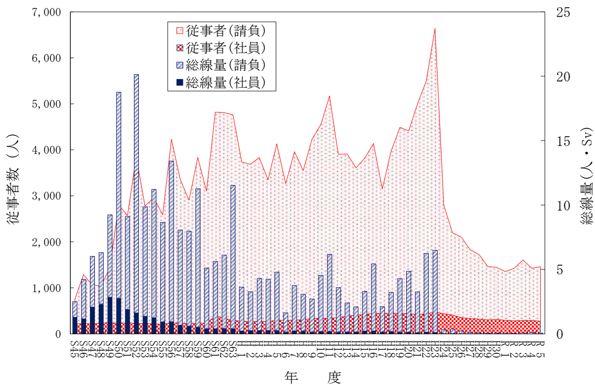
敦賀発電所 従事者数・総線量
