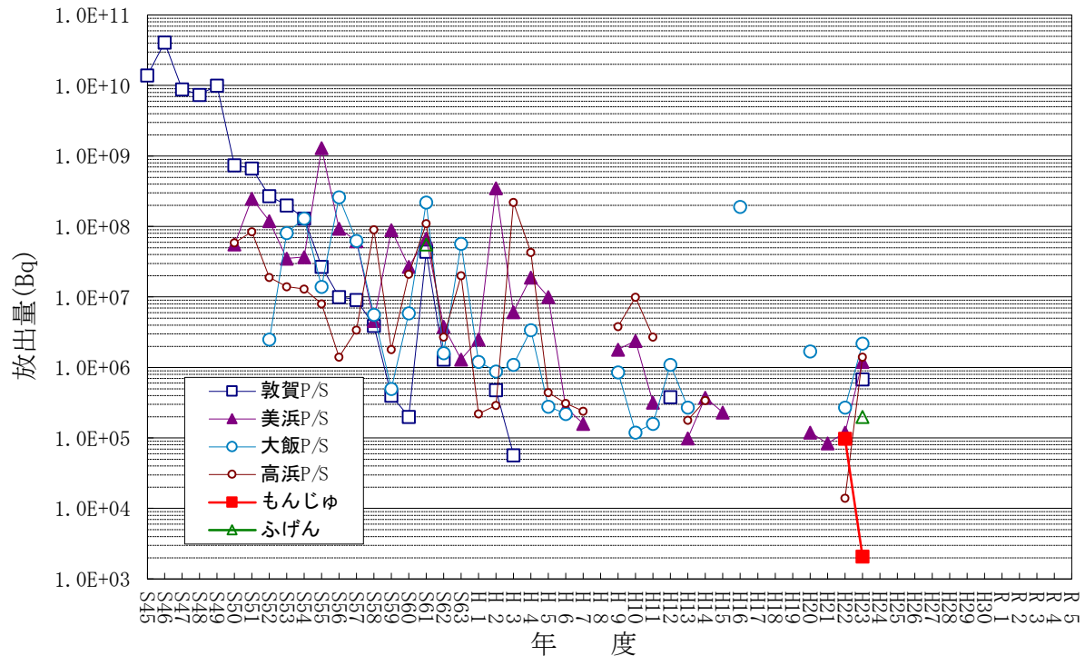
気体廃棄物（ヨウ素 131）放出実績：発電所別
