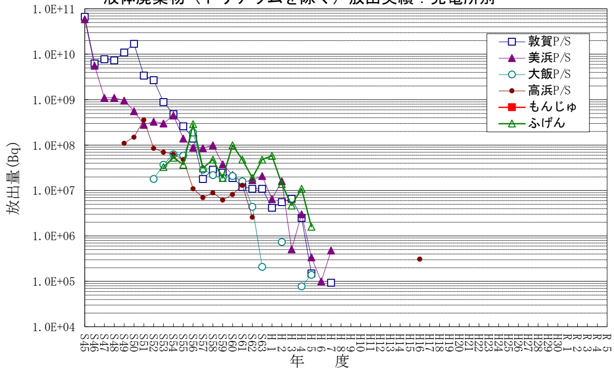
液体廃棄物（トリチウムを除く）放出実績：発電所別
