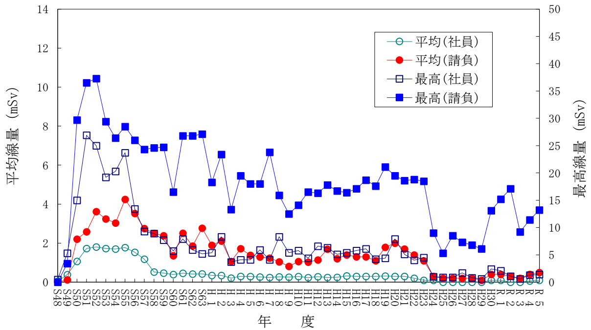
高浜発電所従事者 平均・最高線量
