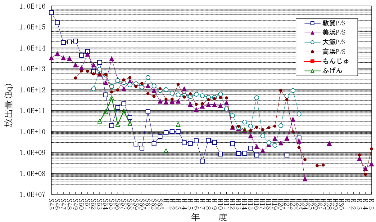
気体廃棄物（希ガス）放出実績：発電所別
