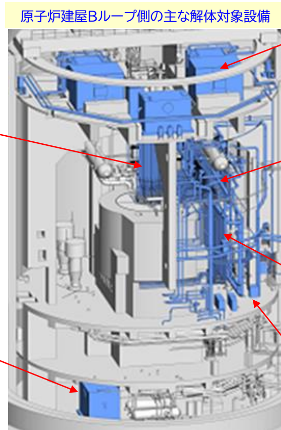
<原子炉建屋内鳥観図>
